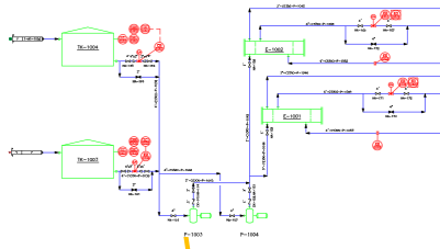
P&ID(配管系統図) 設計 & 関連図書作成
